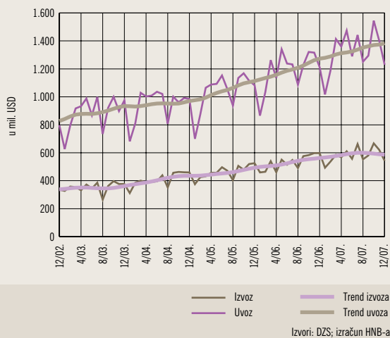
1.60. Robni izvoz (fob) i uvoz (cif) bez ostale transportne opreme te nafte i naftnih derivata po stalnom tečaju iz 2002.
