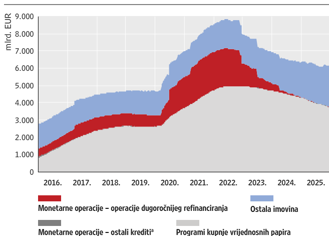
Slika 13. Bilanca Eurosustava
