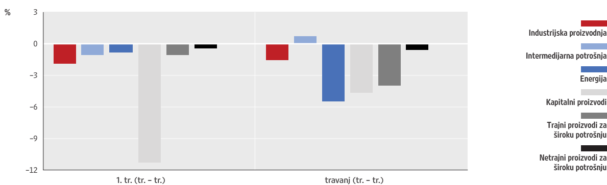
Slika 3.1.7. Industrijska proizvodnja
